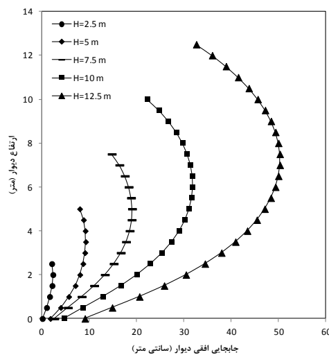
شکل ۱۴. نمودار جابه‌جایی افقی دیوار برای مقادیر مختلف ارتفاع دیوار
