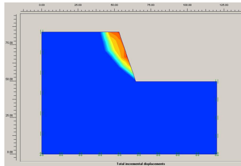
شکل ۳. نمایش تغییرشکل‌های کل برای تحلیل دوبعدی برای ترانشه با ارتفاع ۳۴ متر، شیب ۱ افقی: ۲ قائم و مصالح L1-1
