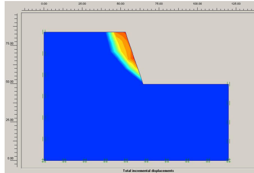
شکل ۳. نمایش تغییرشکل‌های کل برای تحلیل دوبعدی برای ترانشه با ارتفاع ۳۴ متر، شیب ۱ افقی: ۲ قائم و مصالح L1-1
