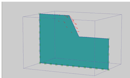
شکل ۳. نمایش تغییرشکل‌های کل برای تحلیل دوبعدی برای ترانشه با ارتفاع ۳۴ متر، شیب ۱ افقی: ۲ قائم و مصالح L1-1
