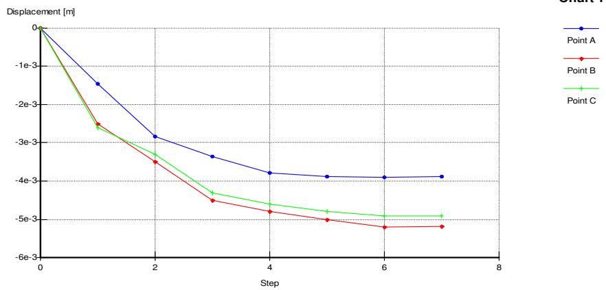
شکل ۱۰. نمودار میزان جاب‌جایی‌های محاسبه شده دیوار و سقف تونل در ایستگاه ۶+۹۶۸ [۴]
