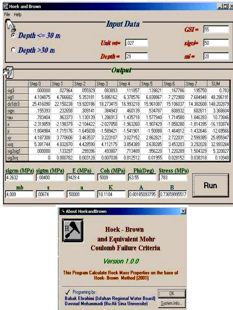
شکل ۴: صفحه اصلی برنامه رایانه‌ای ویژه جهت محاسبه پارامترهای مهندسی توده‌های سنگی
