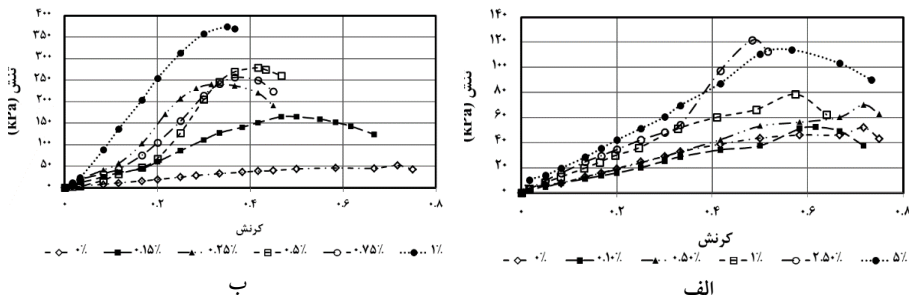
شکل ۷. تاثیر مقادیر مختلف نانوذرات بر مقاومت فشاری محصور نشده خاک بهسازی شده با (الف) نانورس (ب) نانوسیلیکا
