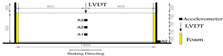
شکل ۲. شکل شماتیک نمونه‌های آزمایش همراه با ابزاربندی جدول ۲. پارامترهای متغیر در آزمایش‌های میز لرزه
