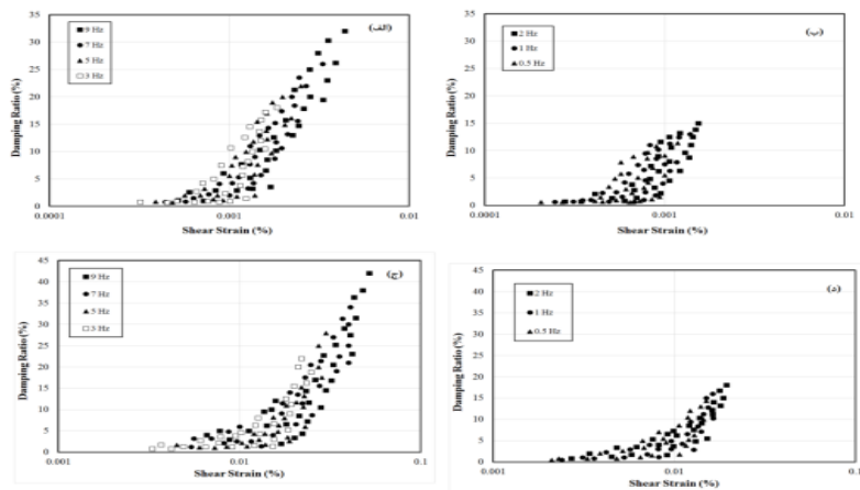
شکل ۲۱. تغییرات نسبت میرایی با کرنش برشی در فرکانس‌های مختلف بارگذاری تحت بارگذاری مستطیلی و شتاب ورودی الف و ب (ب) 0.1g ، ج و د) 0.3g
