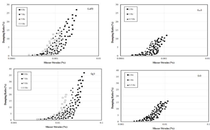
شکل ۲۲. تغییرات نسبت میرایی با کرنش برشی در فرکانس‌های مختلف بارگذاری تحت بارگذاری سینوسی و شتاب ورودی الف و ب (ب) 0.1g ، ج و د) 0.3g
