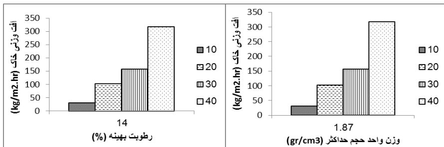
شکل ۱۷. رابطه وزن واحد حجم حداکثر و درصد رطوبت بهینه در مقابل فرسایش‌پذیری لایه میانی
