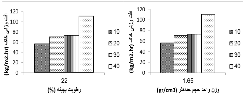
شکل ۱۶. رابطه وزن واحد حجم حداکثر و درصد رطوبت بهینه در مقابل فرسایش‌پذیری
