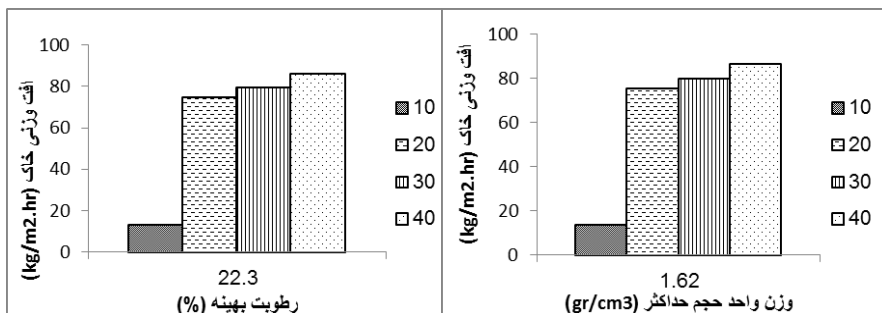
شکل ۱۸. رابطه وزن واحد حجم حداکثر و درصد رطوبت بهینه در مقابل فرسایش‌پذیری لایه پایینی
