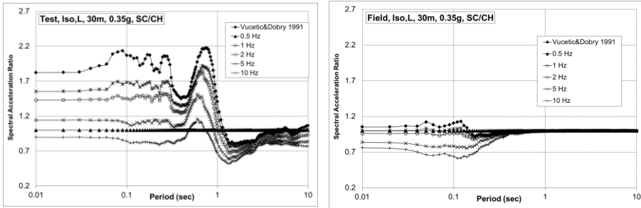
الف) ستون ۳۰ متری خاک نوع I، مینا سرعت موج برشی صحرائی ب) ستون ۳۰ متری خاک نوع IV، مینا سرعت موج برشی آزمایشگاهی شکل ۹. متوسط تغییرات نسبت شتاب طیفی مؤلفه L زلزله‌های میدان نزدیک (PGA=0.35g) به شتاب طیفی مصالح با فرکانس بارگذاری ۰/۵
