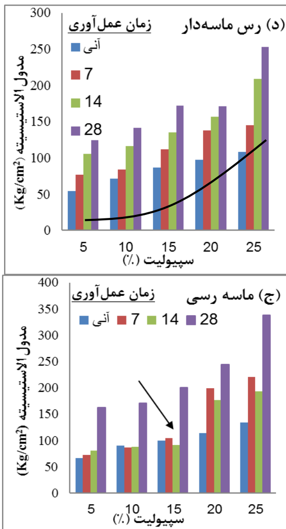
شکل ۵. تغییرات مدول الاستیسیته خاک‌های ماسه رسی (الف و ج) و رس ماسه‌دار (ب و د) تثبیت شده با افزودنی‌های زئولیت (الف و ب) و سیپولیت (ج و د) در درصد و زمان‌های متفاوت عمل‌آوری
