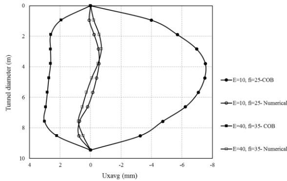
شکل ۵. جابه‌جایی افقی جبهه کار تونل
