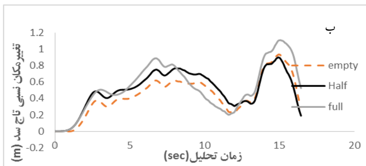
شکل ۹. تغییر مکان نسبی تاج سد در سه حالت خالی، نیمه پر و پر برای زلزله‌های الف) طبس و ب) سانفرناندو
