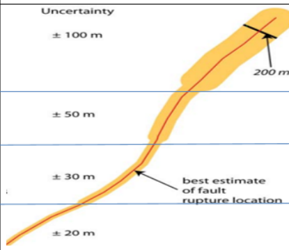
جدول ۶. نمایش حریم گسل و دقت تخمین محدوده گسیختگی در آن، با توجه به سطح اطلاعات موجود [۳۴]، [۳۵]
