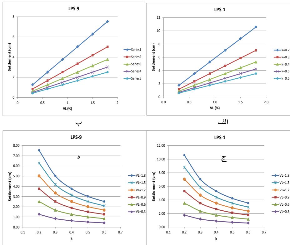
شکل ۱۲. روند تغییرات میزان نشست حداکثر با تغییر پارامترهای k و VL [۱۲]
