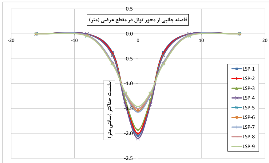
شکل ۶. منحنی‌های گودی نشست (پیش‌بینی شده) در مقاطع عرضی برای نقاط بررسی شده [۱] و جدول ۷. ارزیابی نشست به روش تحلیلی لگاناتان و پولوس [۲۲] با فرض g=0.019 \text{ m}
