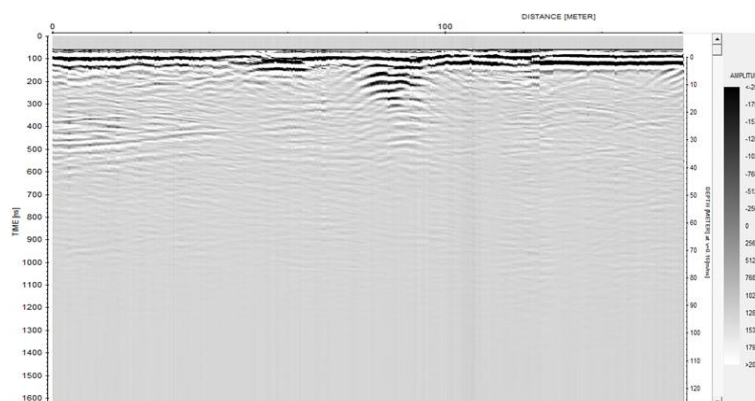
شکل ۴. نداشت راداری داده‌های خام GPR در منطقه علم‌کوه
