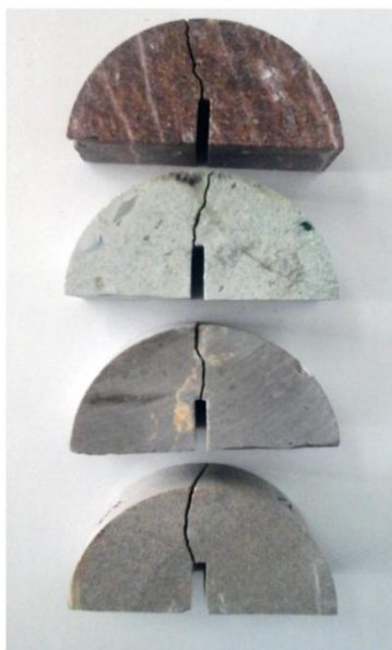
شکل ۳. نمونه‌ها بعد از آزمایش برای نوع سنگ ۴ (از بالا به پایین آندزیت، توف سبز، سنگ آهک و ماسه سنگ)
