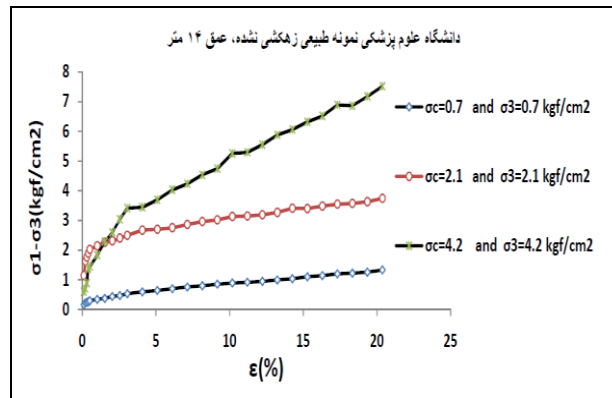
شکل ۲۲. منحنی‌های تنش- کرنش محوری نمونه‌های طبیعی زهکشی نشده، دانشگاه علوم پزشکی کرمان عمق ۱۴-۱۶ متر
