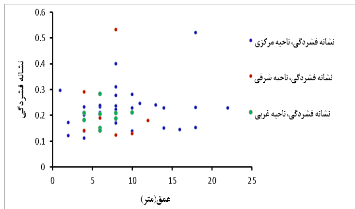
شکل ۸. رابطه نشانه فشردگی با عمق در نواحی سه‌گانه در محدوده شهر کرمان
