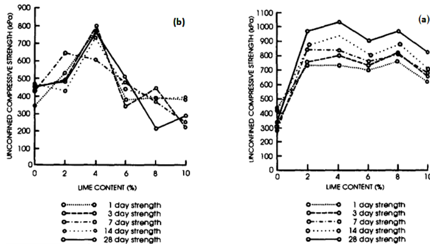
شکل ۱. مقاومت فشاری ساده: (a) کائولینیت، (b) مونتوریلونیت با درصدهای مختلف آهک [۸]
