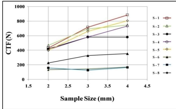
شکل ۸. مقایسه میانگین مقادیر CTF مربوط به خرده ذرات در اندازه‌های مختلف که با نفوذکننده ۰/۸ میلی‌متری آزمایش شده‌اند
